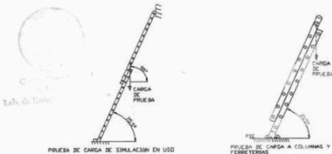
Fig. 2. Prueba de carga inclinada y prueba de carga a columnas y ferretería
