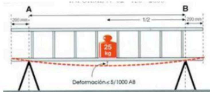
Ensayo a flexión lateral
