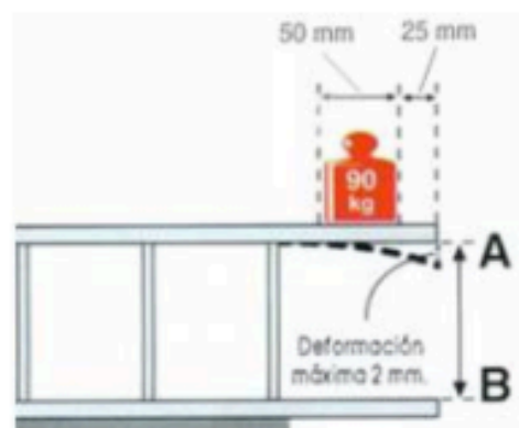
Ensayo Resistencia Extremidades Se probaron todos los perfiles con resultados satisfactorios Señalando una deformación menor de la permitida
